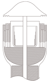
III Klammernahltreihen Senkkopftechnologie
